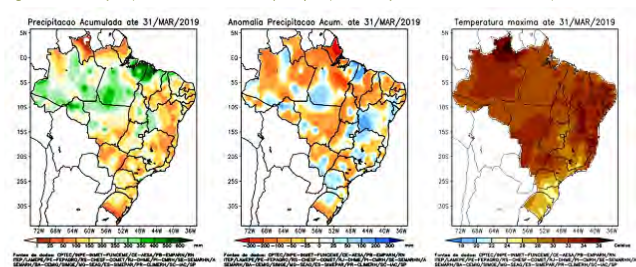
Figura 24 – Precipitação total, anomalia de precipitação e temperatura máxima em março de 2019
