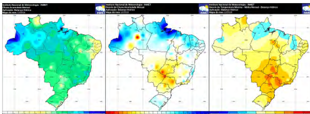
Figura 2 – Precipitação total, desvio da precipitação e desvio da temperatura máxima, em relação à média histórica, nos meses com maiores restrições no desenvolvimento da safra 2019/20 na Região Centro-Sul e no sul da Bahia - Dezembro 2018
