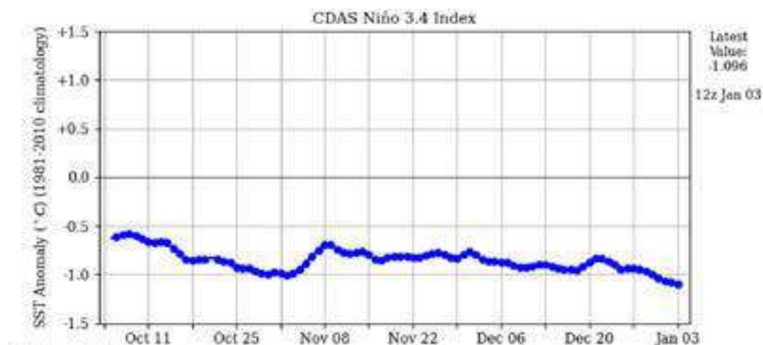
GRÁFICO 1 - DE MONITORAMENTO DO ÍNDICE DIÁRIO DE EL NIÑO/LA NIÑA NA REGIÃO 3.4
