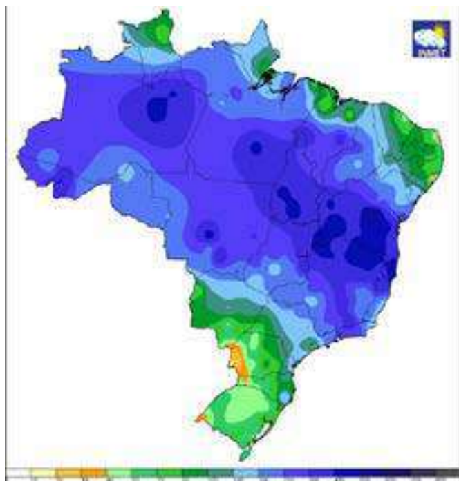
FIGURA 1 - MAPA DE PRECIPITAÇÃO ACUMULADA EM DEZEMBRO DE 2021
