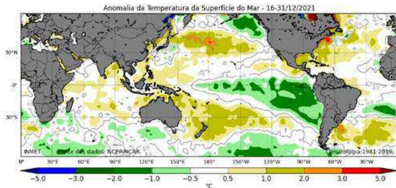
FIGURA 2 - MAPA DE ANOMALIAS DA TSM NO PERÍODO DE 16 A 31/12/2021
