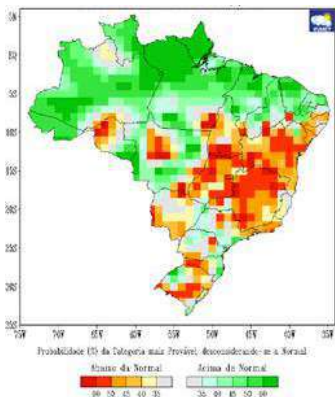
FIGURA 3 - PREVISÃO PROBABILÍSTICA DE PRECIPITAÇÃO PARA O TRIMESTRE JANEIRO/2021 E FEVEREIRO-MARÇO/2022
