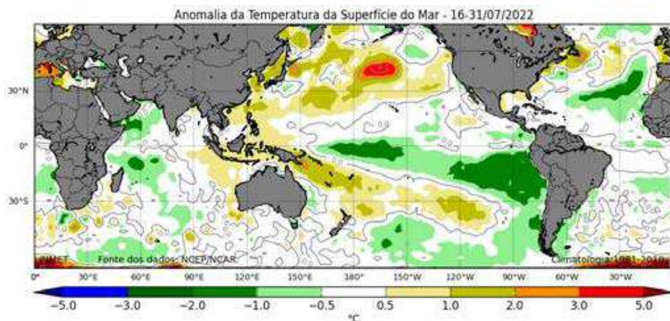
FIGURA 2 - MAPA DE ANOMALIAS DA TSM NO PERÍODO DE 16 A 31 DE JULHO/JULHO/2022
