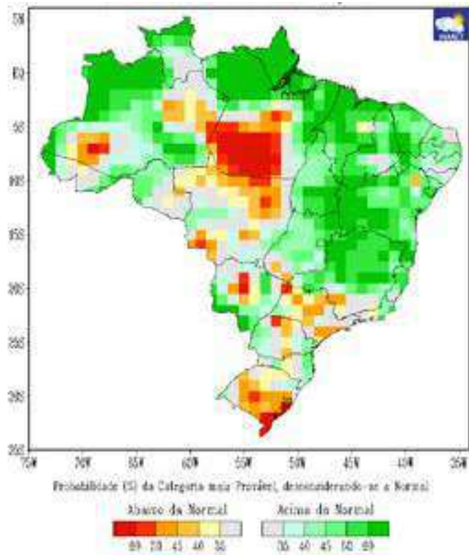
FIGURA 3 - PREVISÃO PROBABILÍSTICA DE PRECIPITAÇÃO PARA O TRIMESTRE AGOSTO-SETEMBRO-OUTUBRO DE 2022
